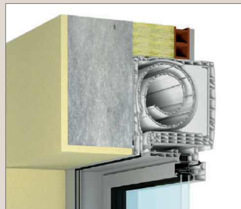
Le bloc-baie Thermobloc
