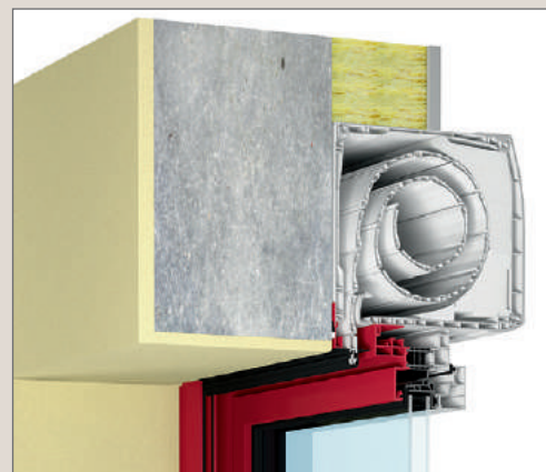
Le bloc-baie Classic
