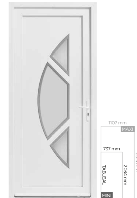
CYCLONE Vitrage feuilleté sablé affleurant, décors aspect inox. Ud = 1,8
