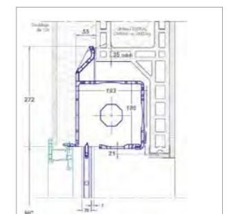
Schéma volet roulant demi-linteau.
