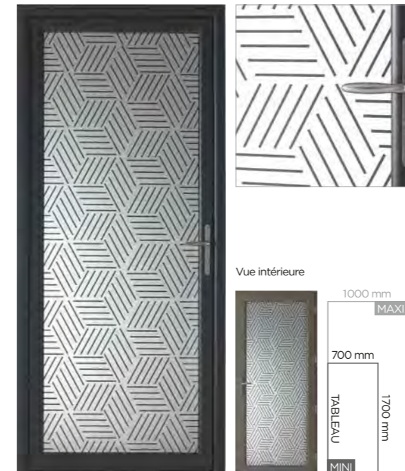
BONITE Décors laqués noirs à l'intérieur du vitrage feuilleté. Ud = 1,5
