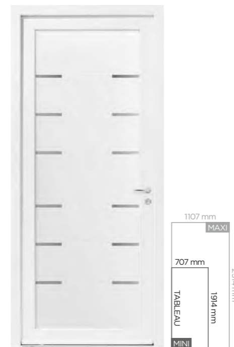
BRÉHAT Design exclusif. Porte rainurée 2 faces. Ud = 1,6
