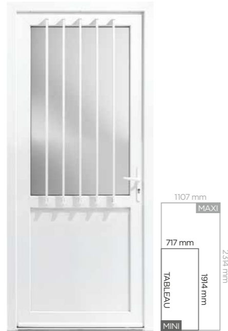
PECARI Double vitrage feuilleté sablé et barreaudage aluminium. Ud = 1,4
