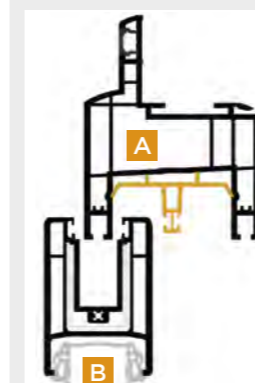
COUPE VERTICALE
