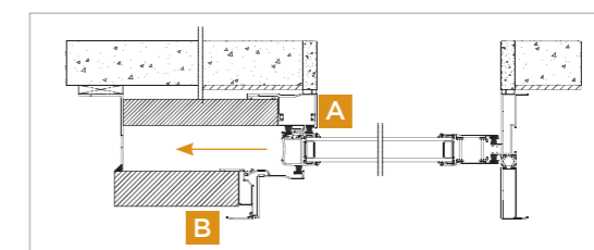
Galandage 1 rail 1 vantail ou 2 rails 2 vantaux. Option cadre dormant isolé prêt à poser. Possibilité d'encastrement 30 mm. Largeur de passage tableau : - avec VR : -99,5 mm - sans VR : -68,5 mm
