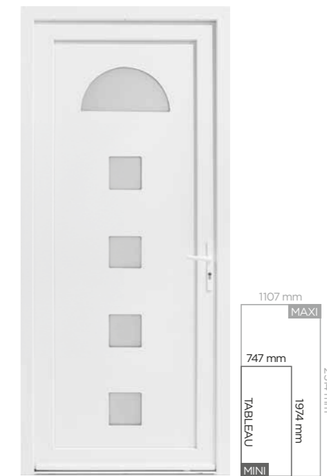
EGOA Vitrage feuilleté sablé affleurant, décors aspect inox en option. Ud = 1,7
