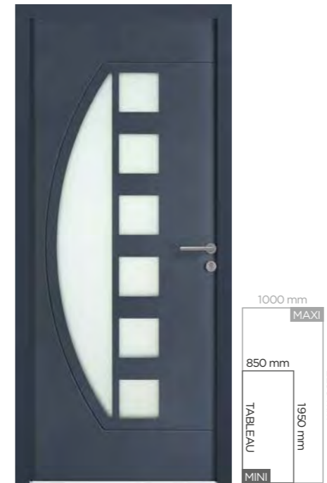
PARTY 60 MM Rainuré 2 faces avec triple vitrage feuilleté sablé affleurant. Ud = 1,3
