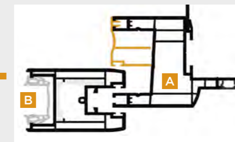
COUPE HORIZONTALE
