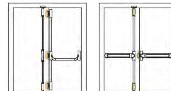
Barre anti-panique 1 point ou 3 points de fermeture + crémone pompier sur semi-fixe.
