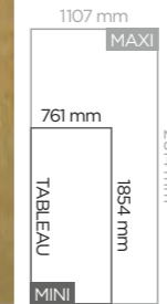
CITELLE Plaxé chêne irlandais (en option), vitrage delta clair avec petits-bois incorporés aspect laiton. Ud = 1,7
