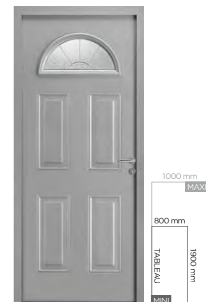
SOLA 60 MM Ouvrant post-formé 2 faces et petits-bois intégrés aspect plomb. Ud = 1,2
