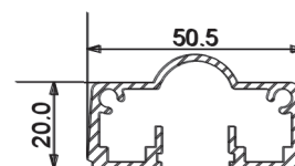
● LISSE TÊTE DE POTEAU GC4022N
