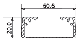
■ LISSE TÊTE DE POTEAU GC4021N
