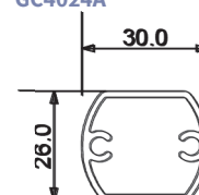
● LISSE INTERMÉDIAIRE GC4024A
